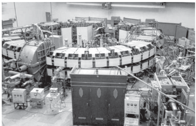
Вид ускорителя «ПАХРА»
