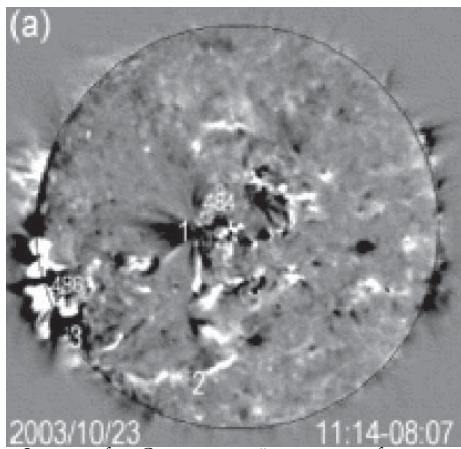
2003/10/23 11:14:08:07 Фотография Солнца в крайнем ультрафиолете, линия 175 А, со спутника КОРОНАС-Ф, полученная 23 октября 2003 года
